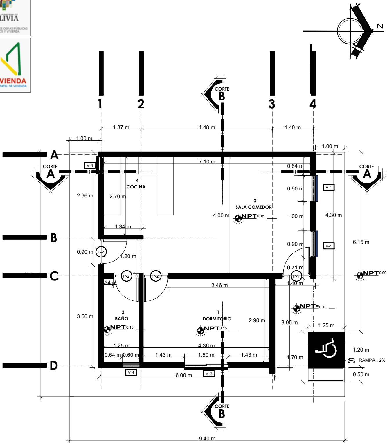
PLANO DE PLANTA ACOTADA
