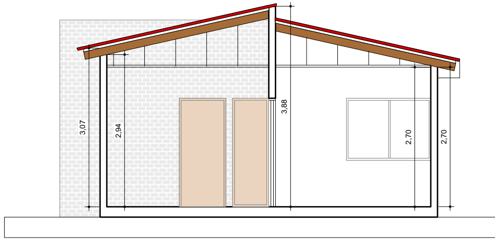
12 CORTES Scale: 1:75
