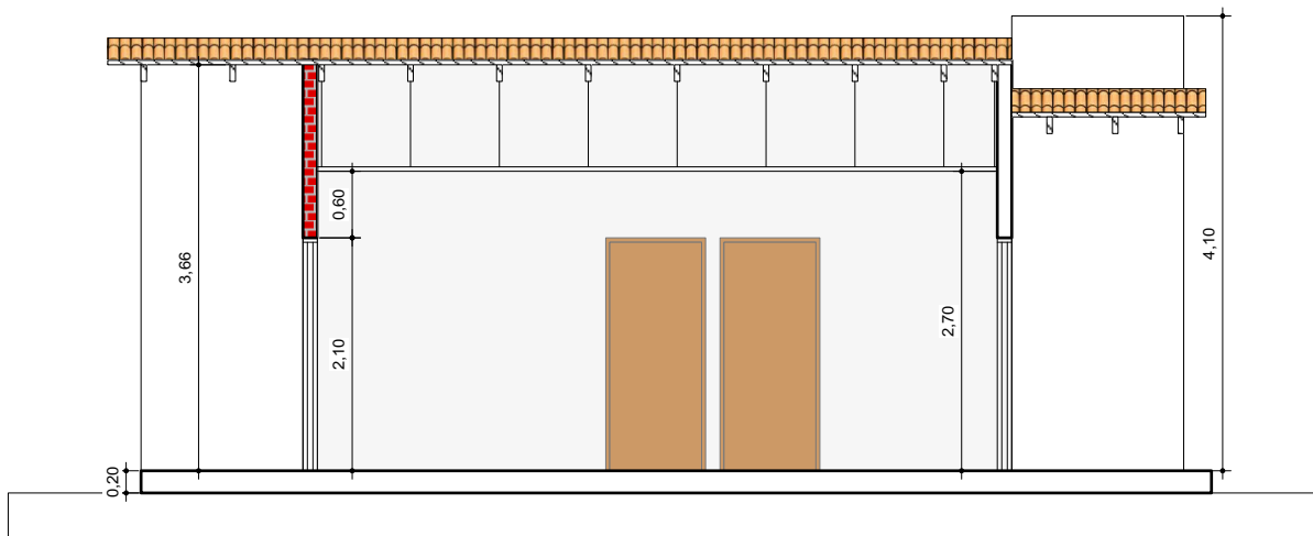
13 CORTES Scale: 1:75
