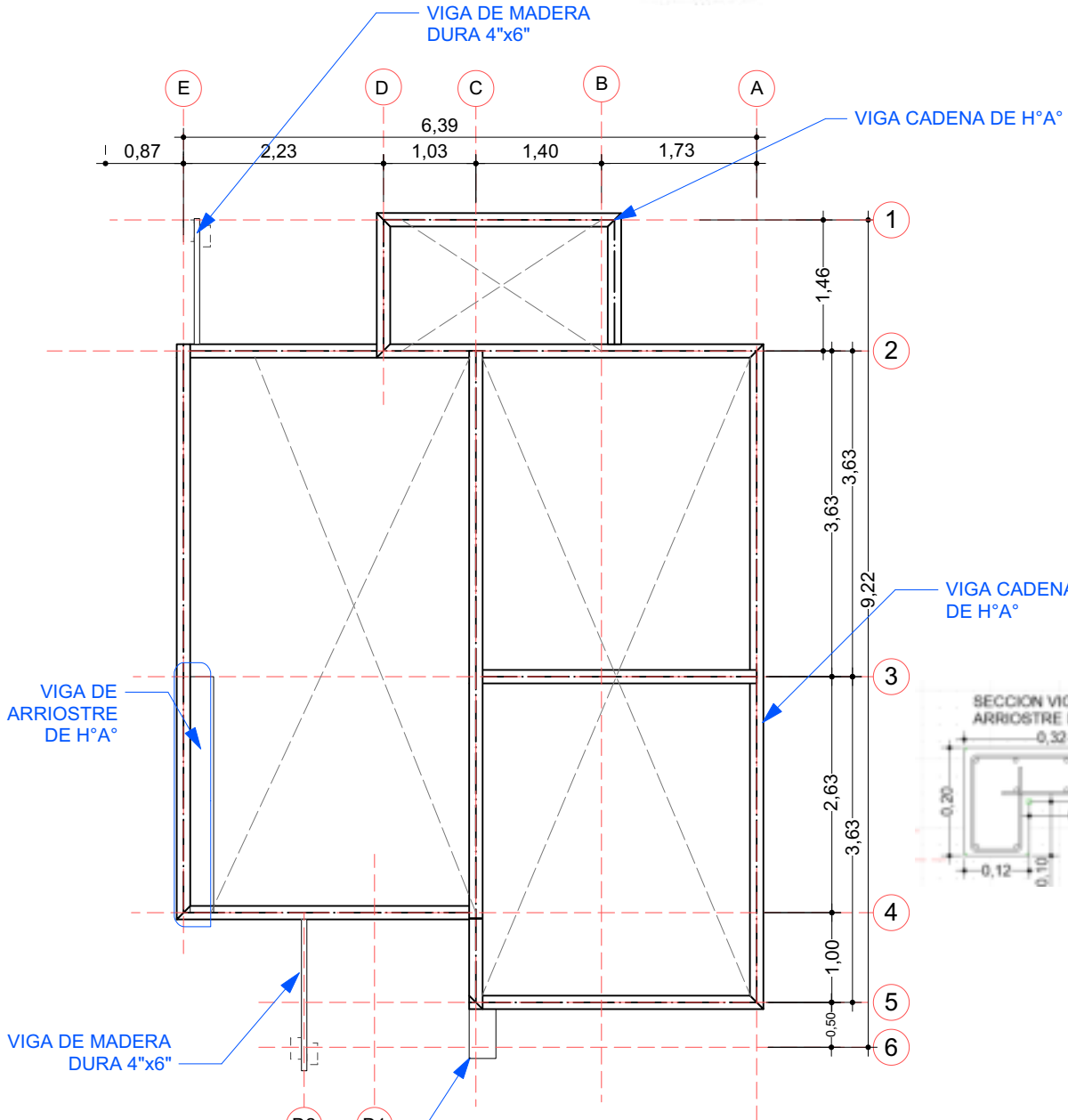
4 PLANO DE VIGA ENCADENADO Scale: 1:75
