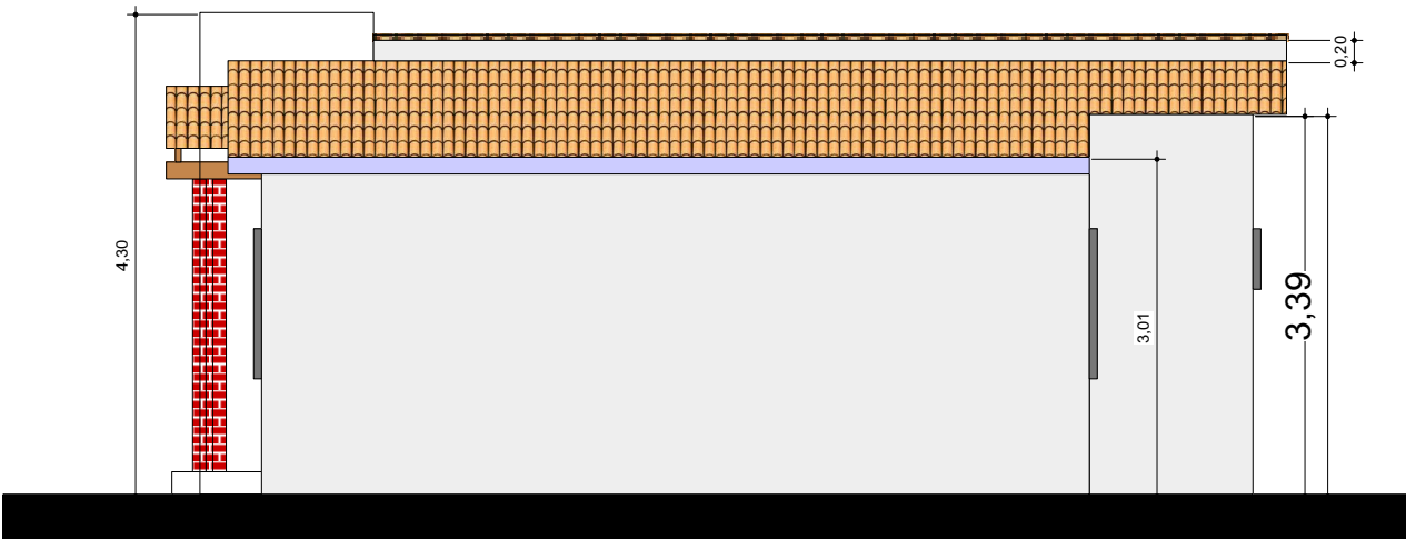
FACHADAS Scale: 1:75
