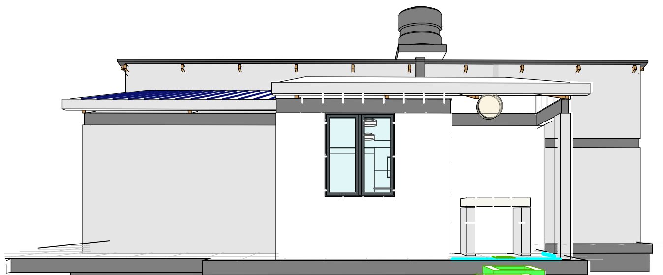
2 PERSPECTIVA LATERAL IZQUIERDO AR-09
