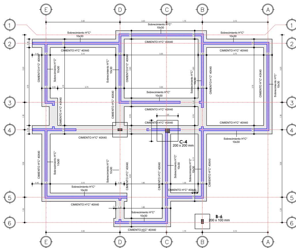
1 PLANO DE CIMIENTOS AR-01 1 : 100
