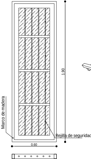
Ventana Tipo 4
