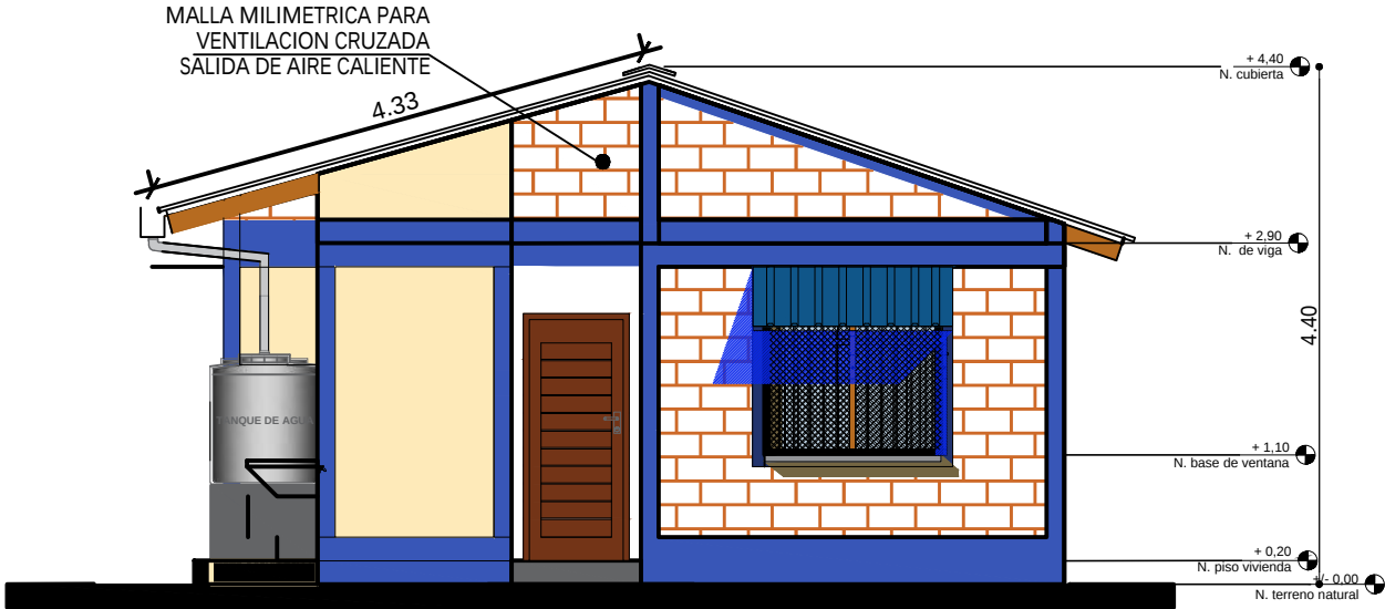
ELEVACION POSTERIOR SC. 1:75
