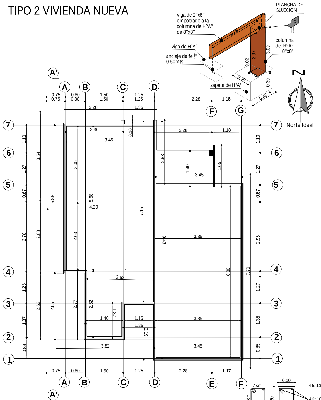
PLANO VIGA CADENA DE H°A° ESC. 1:75
