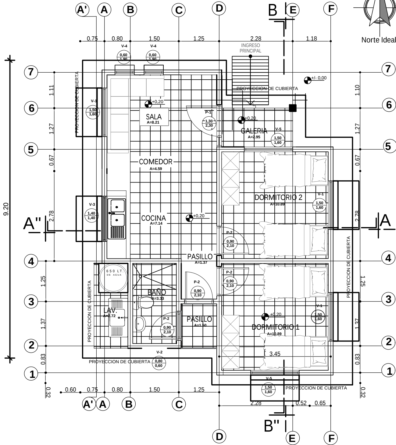
PLANTA AMOBLADA ESC. 1:75
