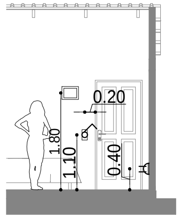
DETALLE ALTURA DE TOMACORRIENTES /INTERRUPTORES
