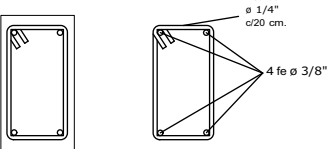
SECCION VIGA CADENA DE H'A°
