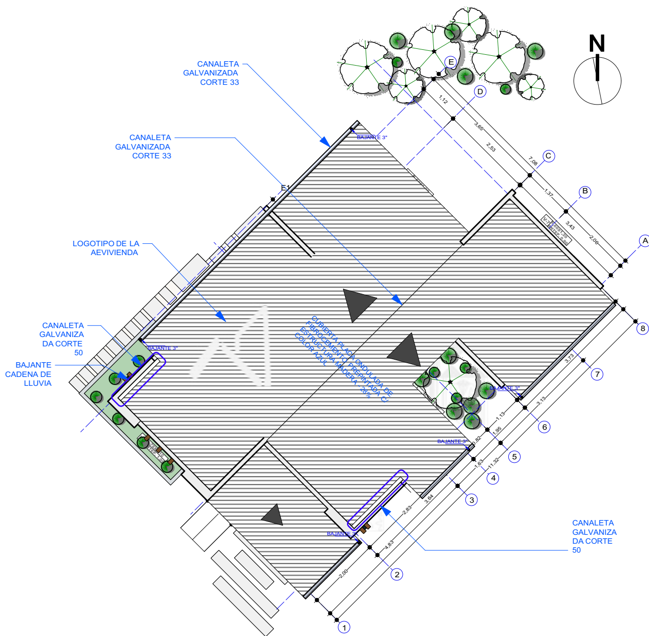
7 PLANO DE CUBIERTA Scale: 1:100
