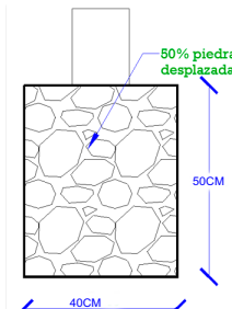
BASE DE HORMIGON CICLOPEO PARA COLUMNA
