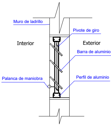
SECCION A-A
