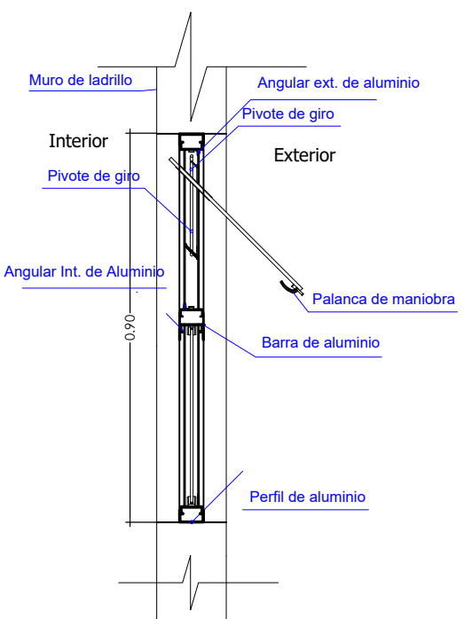
SECCION A-A
