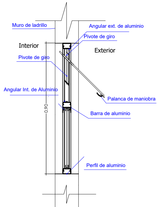
SECCION A-A
