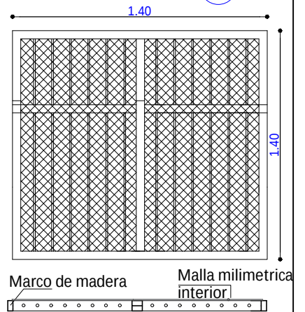
Ventana Tipo 3
