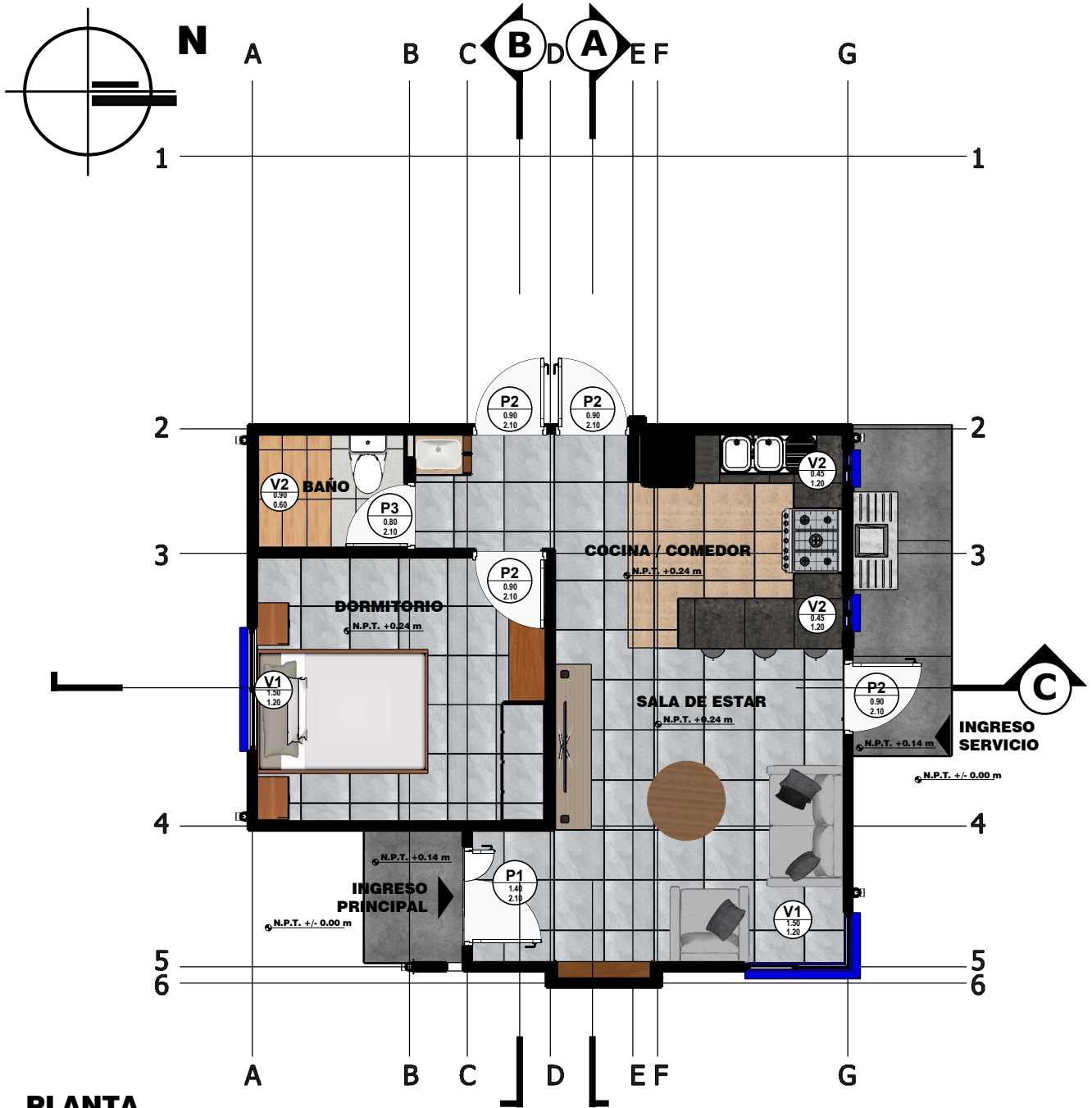
PLANTA ESC. 1:75
