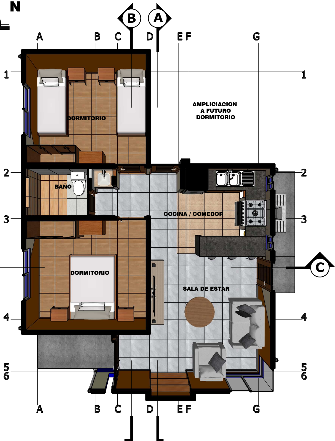
PLANTA FUGADA ESC. 1:75
