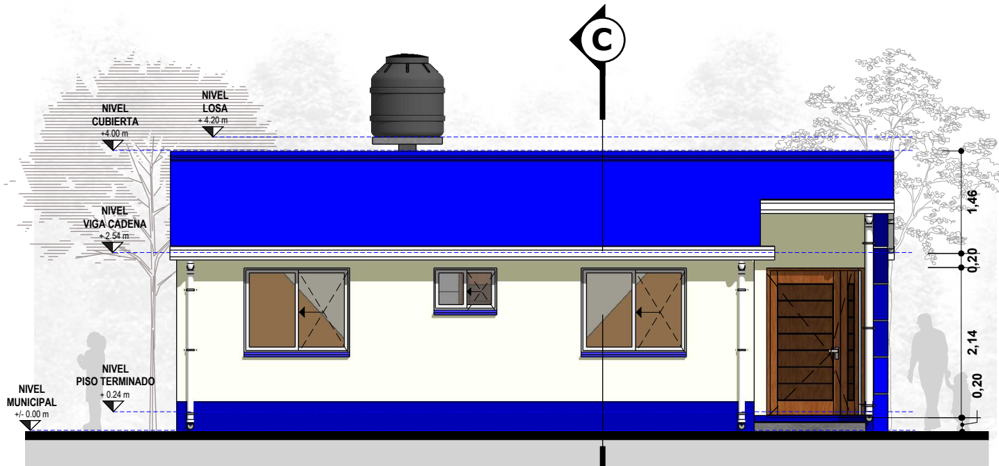
LATERAL ESC. 1:75
